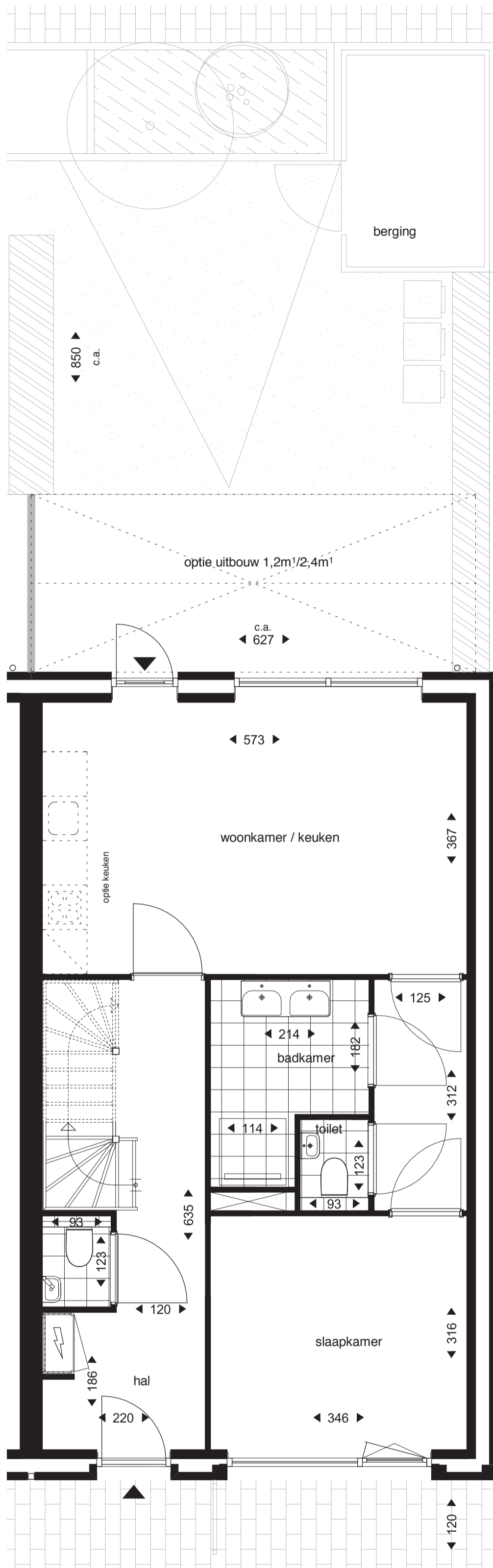
Begane grond
