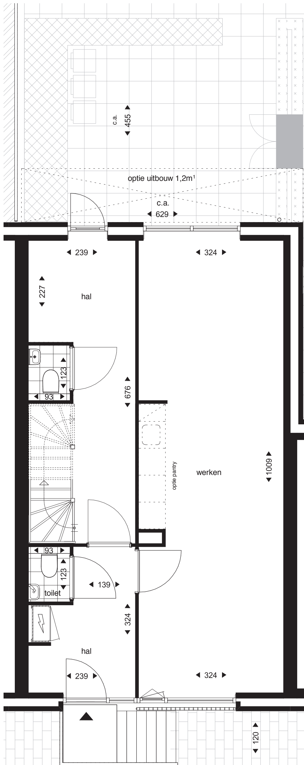
Begane grond
