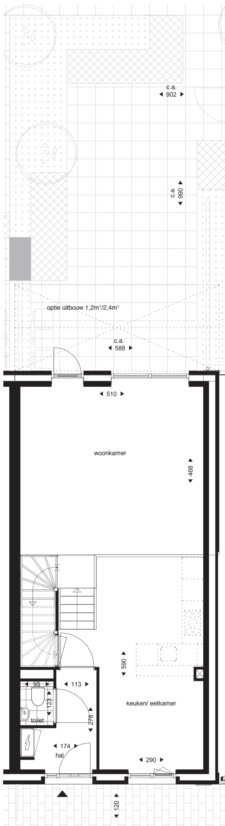
Begane grond
